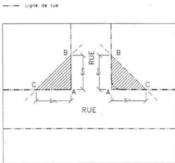
Figure 2.7e : Triangle de visibilité
